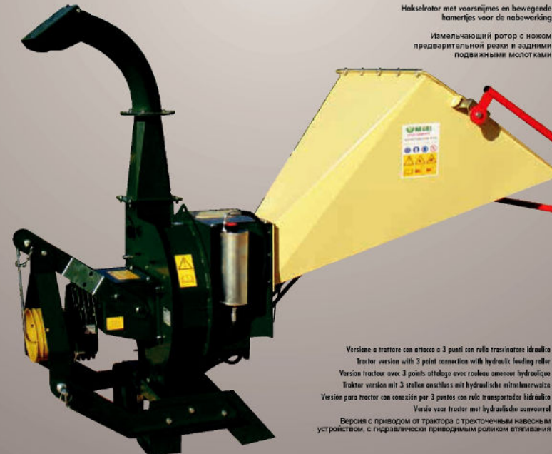
Häckselsystem mit Vorschneidmesser und beweglicher Klingen
